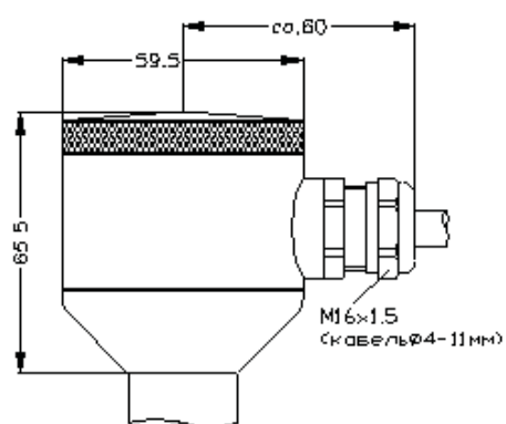
Полевач корпус Каб B00 (IP67)
